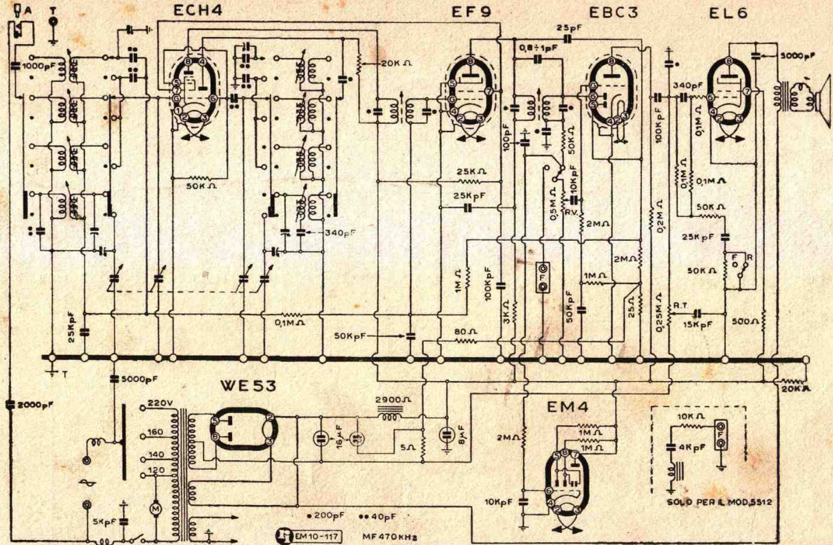
Lo schema elettrico del Phonola 5511 - 5512
